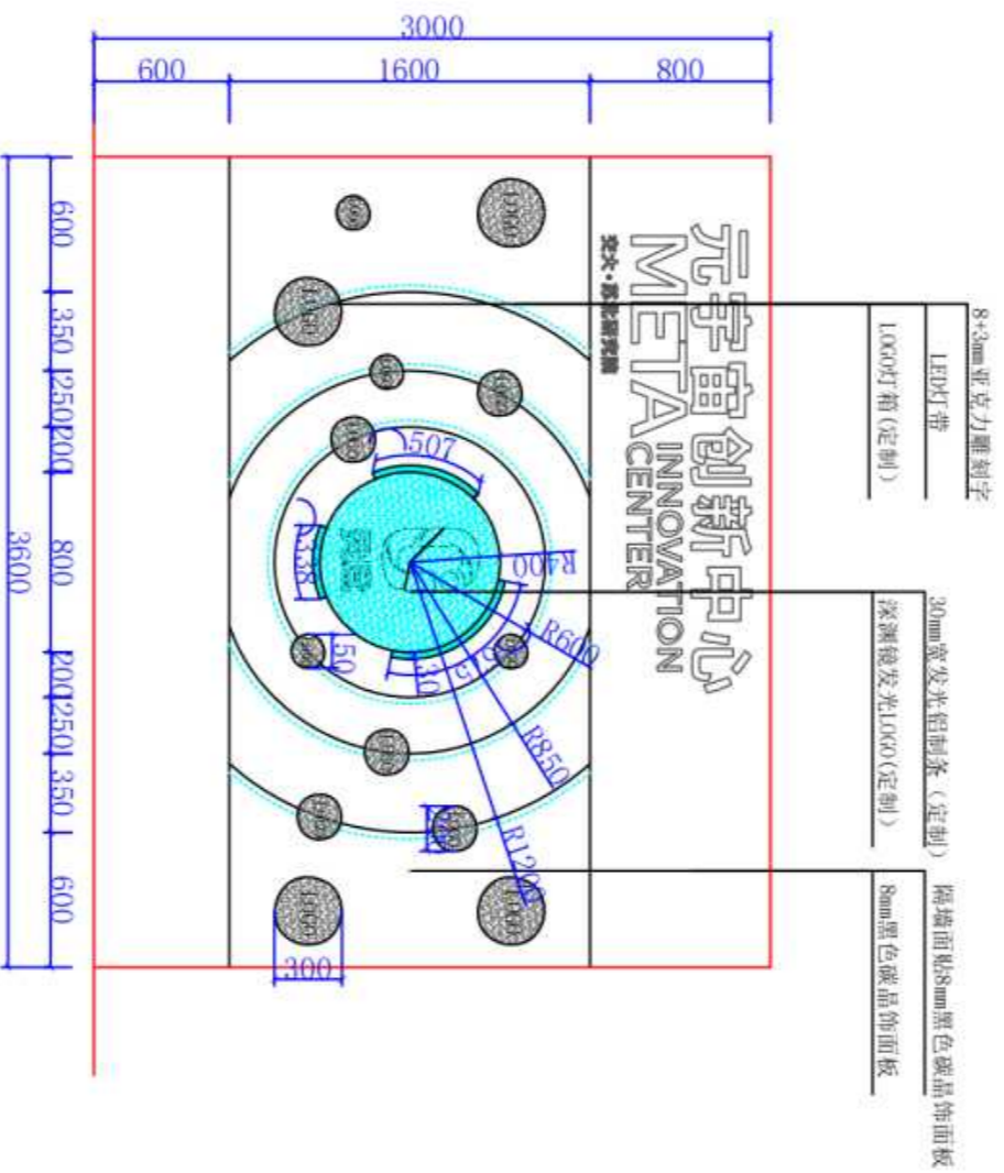
A立面图
