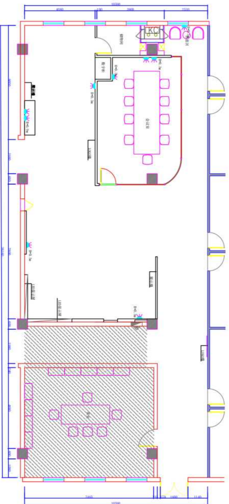
插座布置图
